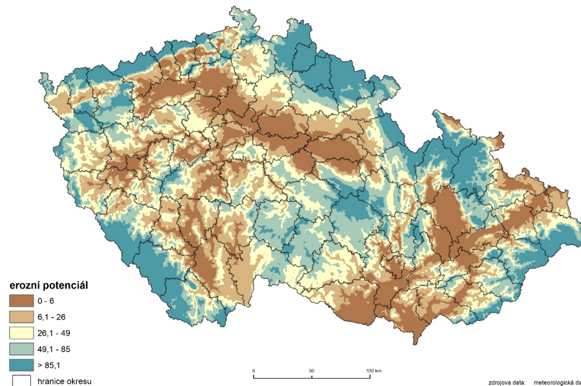
Mapa erozního potenciálu zpracovaného z dat za normálové období 1991-2020
